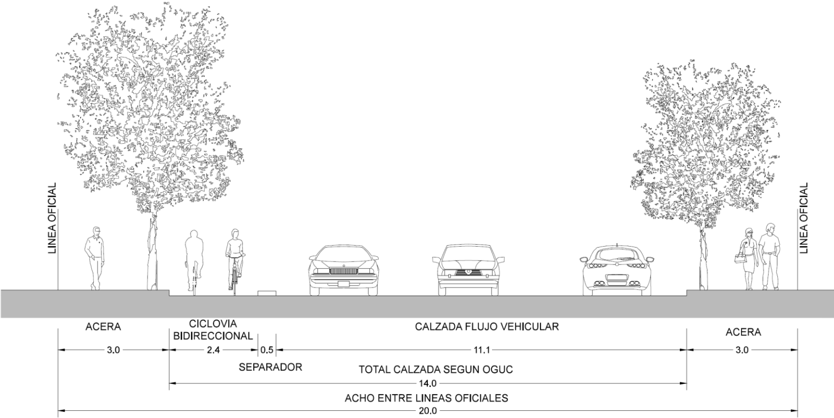
Figura 5 Perfil propuesto Vías Colectoras, que incorpora Ciclovía
