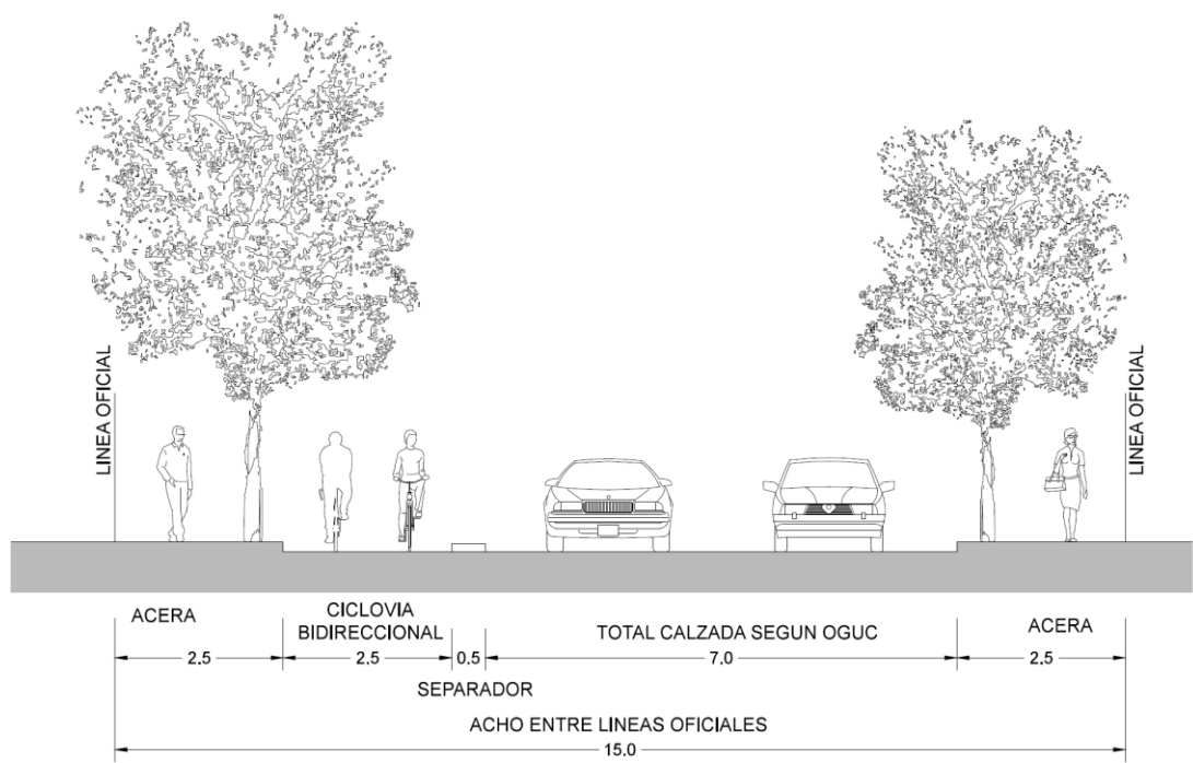
Figura 6 Perfil Propuesto Vías de Servicio
